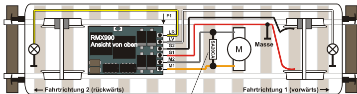
Schutzdiode SA20CA für Fahrzeuge H0 und grösser
